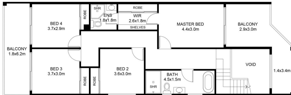
F I R S T F L O O R
